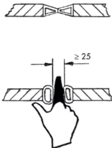
Bild 10: Sicherheitsabstand nach Verformung von Dichtleisten
