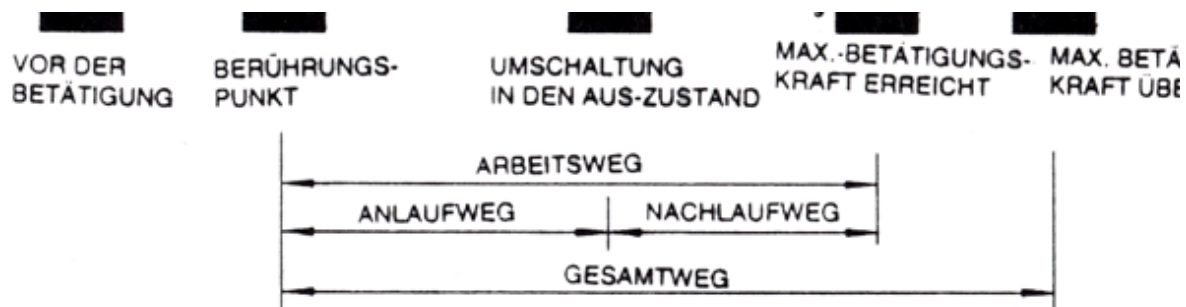
Bild 6: Kraft-Weg-Verlauf einer Schaltleiste
