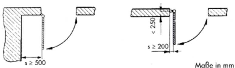
Bild 14: Sicherheitsabstände an Drehflügeltoren
