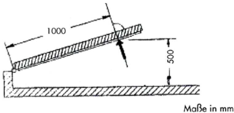
Bild 15: Kraftbegrenzung zwischen Flügel und Umgebung
