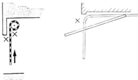
Bild 16: Einzugsstellen im Bereich des Sturzes
