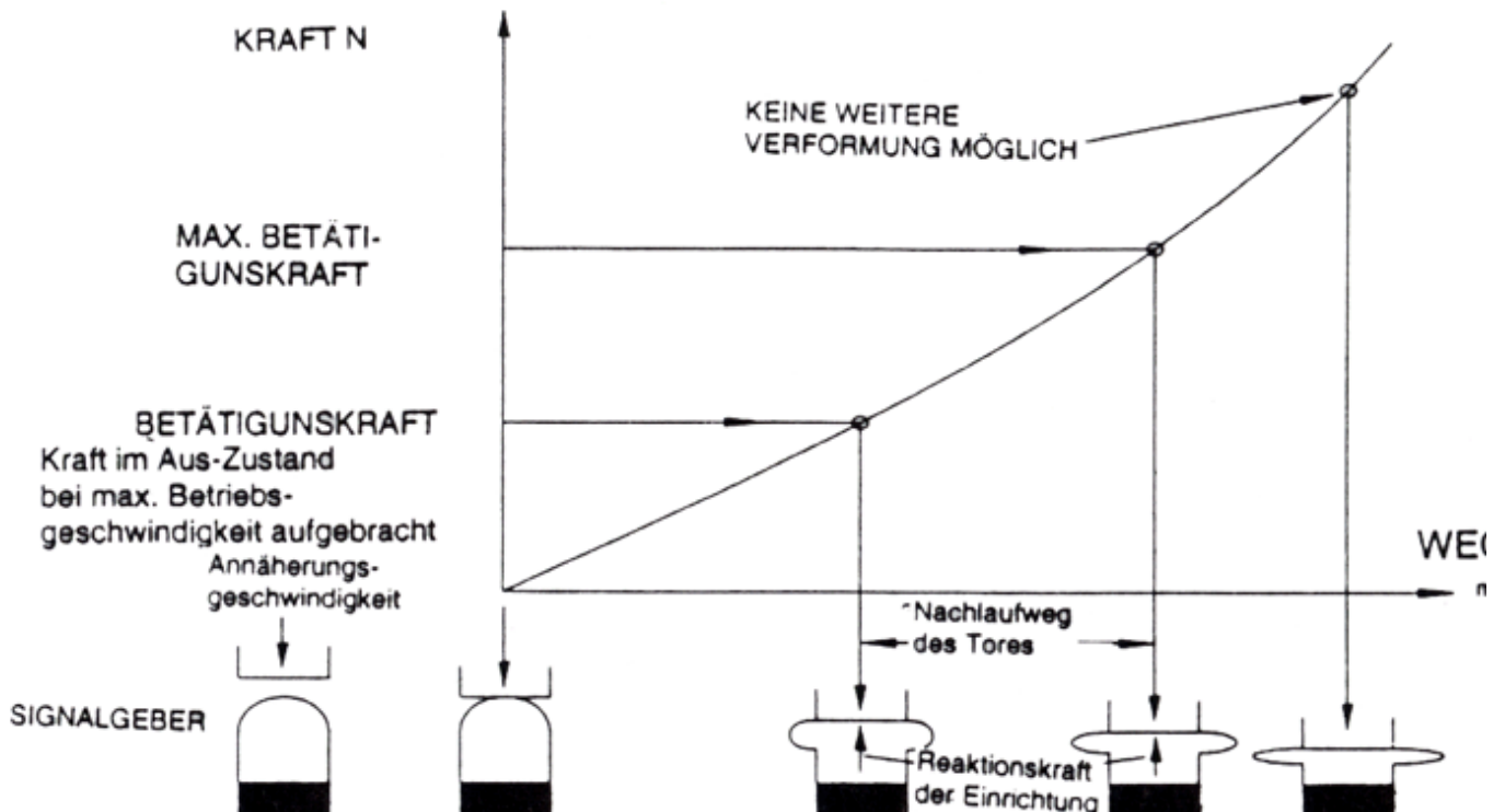
Bild 5: Anordnung einer Schaltleiste
