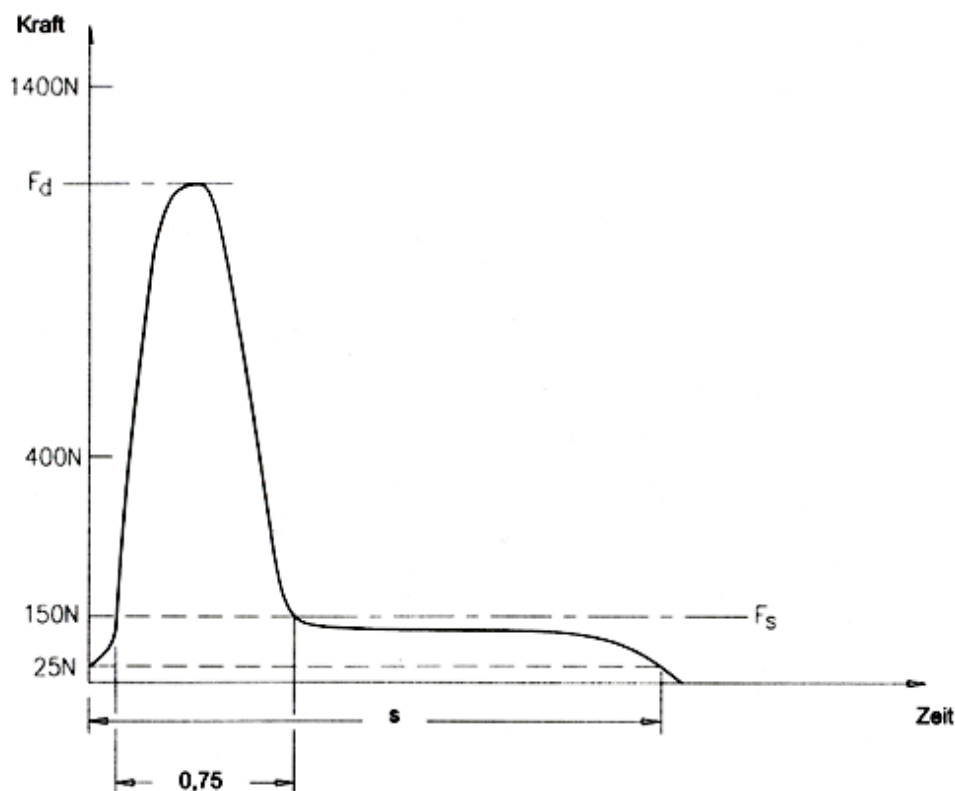
Bild 7: Prinzipdarstellung: Schließkraft in Abhängigkeit der Zeit
